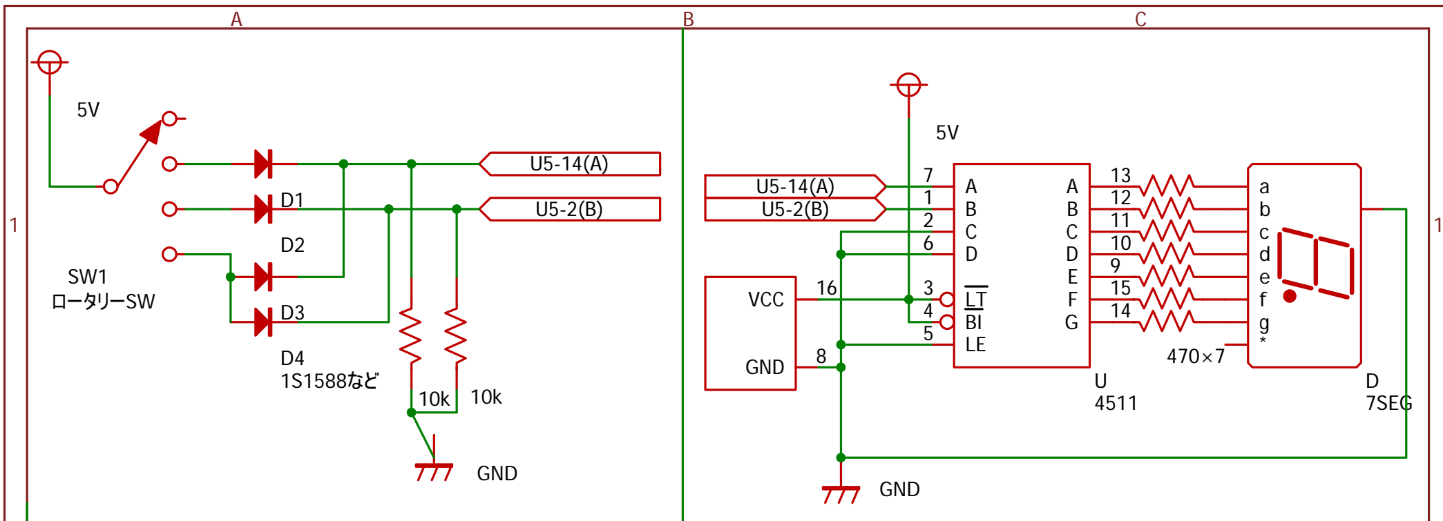
ダイオードマトリクスによるセレクト
