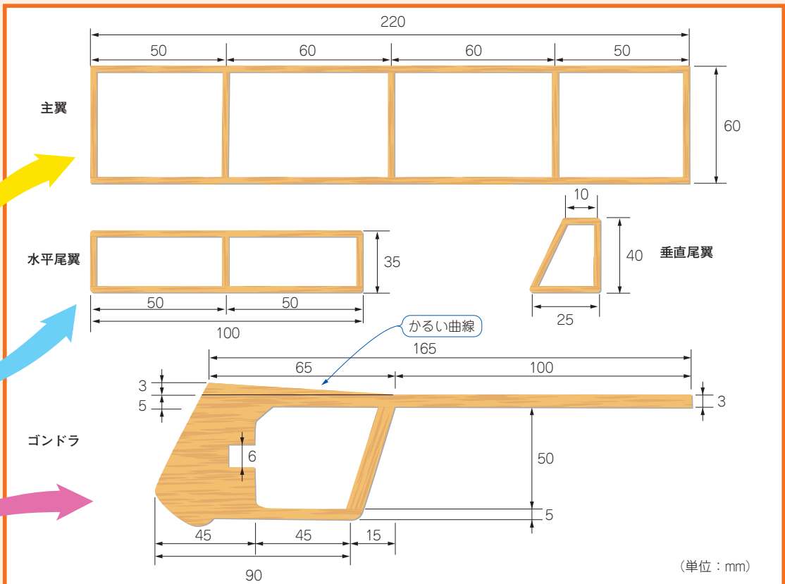
機体の部品展開図
