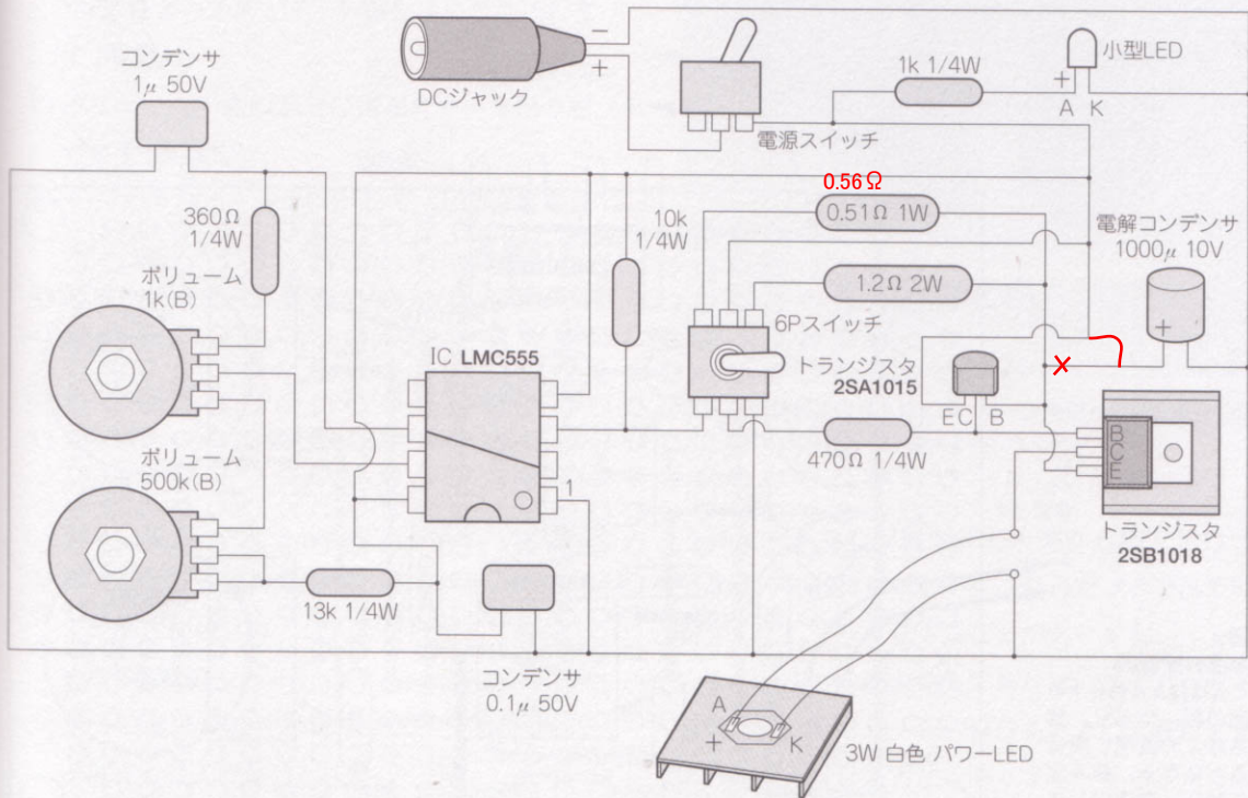
図1 本ストロボ装置の回路図
